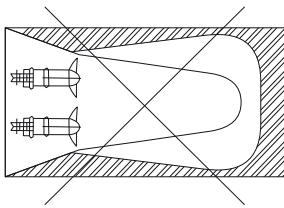
利用池壁反射 Use wall reflections
